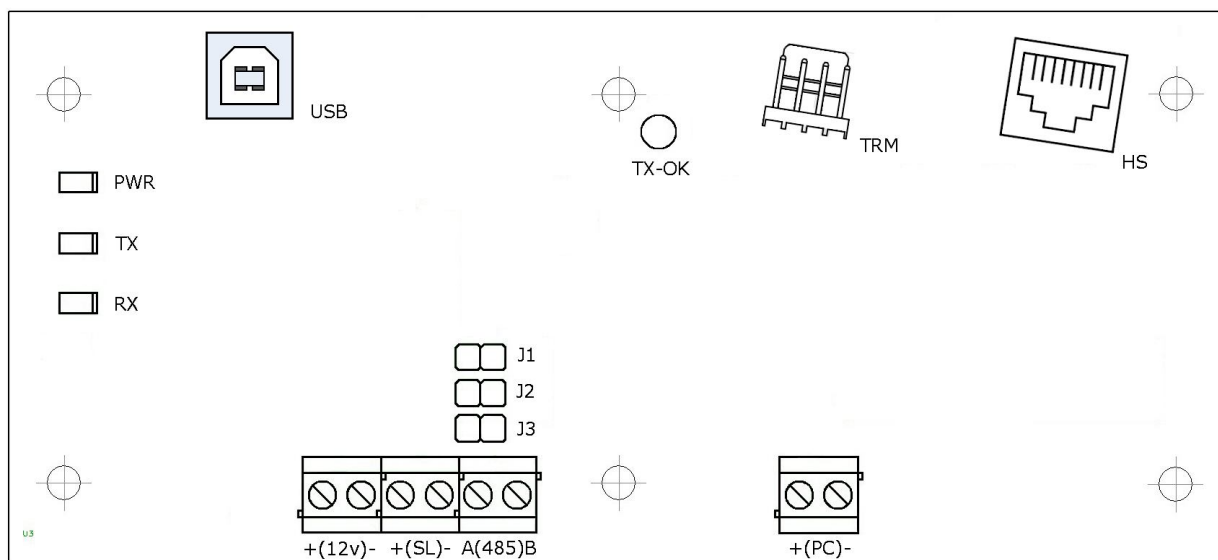
Рисунок 1. Плата MP-251W1
